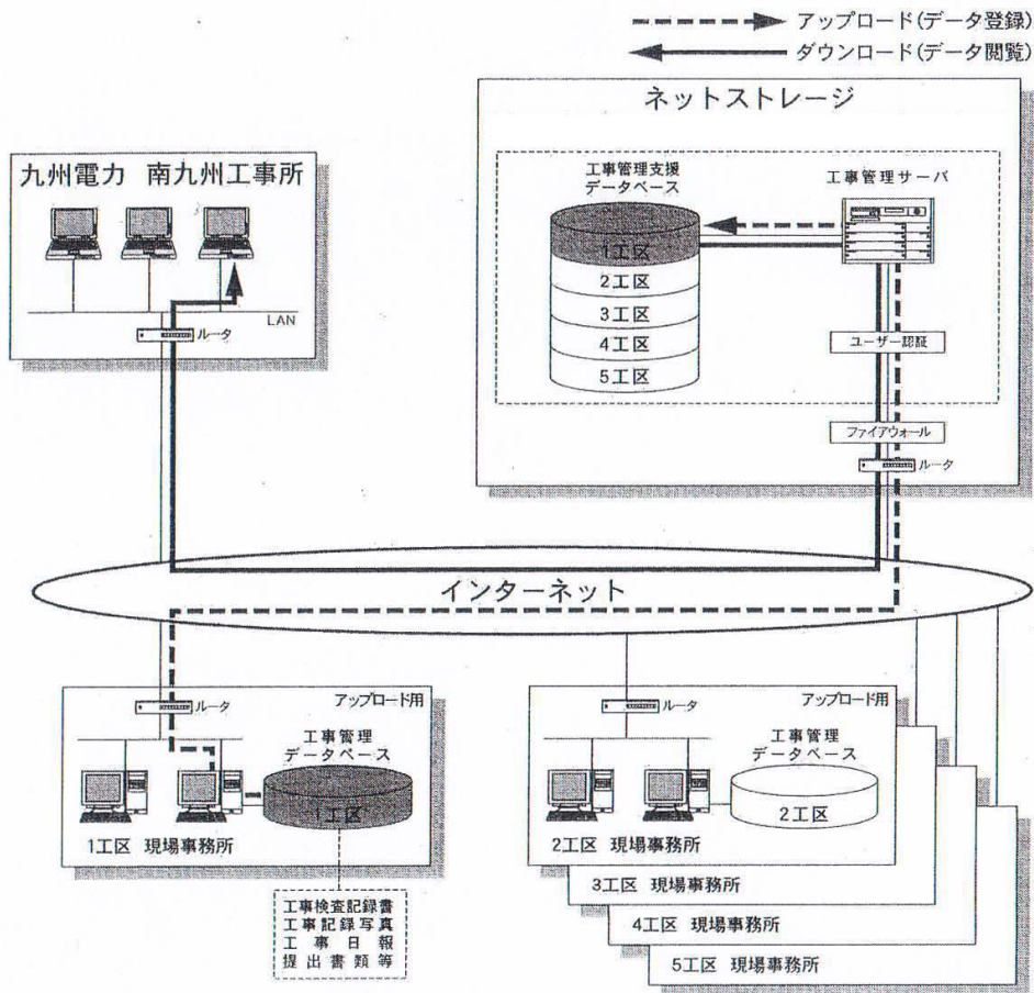
第6図 工事関連支援システム概要図
